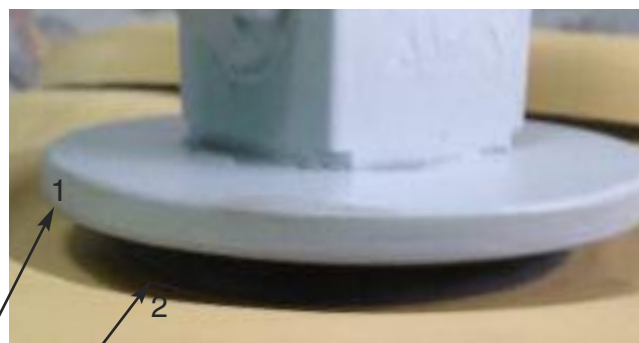
1) RONDELLE \varnothing 120 , épaisseur 8mm 2) SILENTBLOC SUPÉRIEUR)
