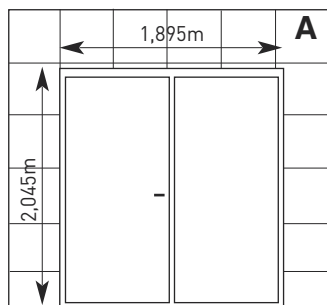
Porte-fenêtre
