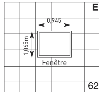
Fenêtre
